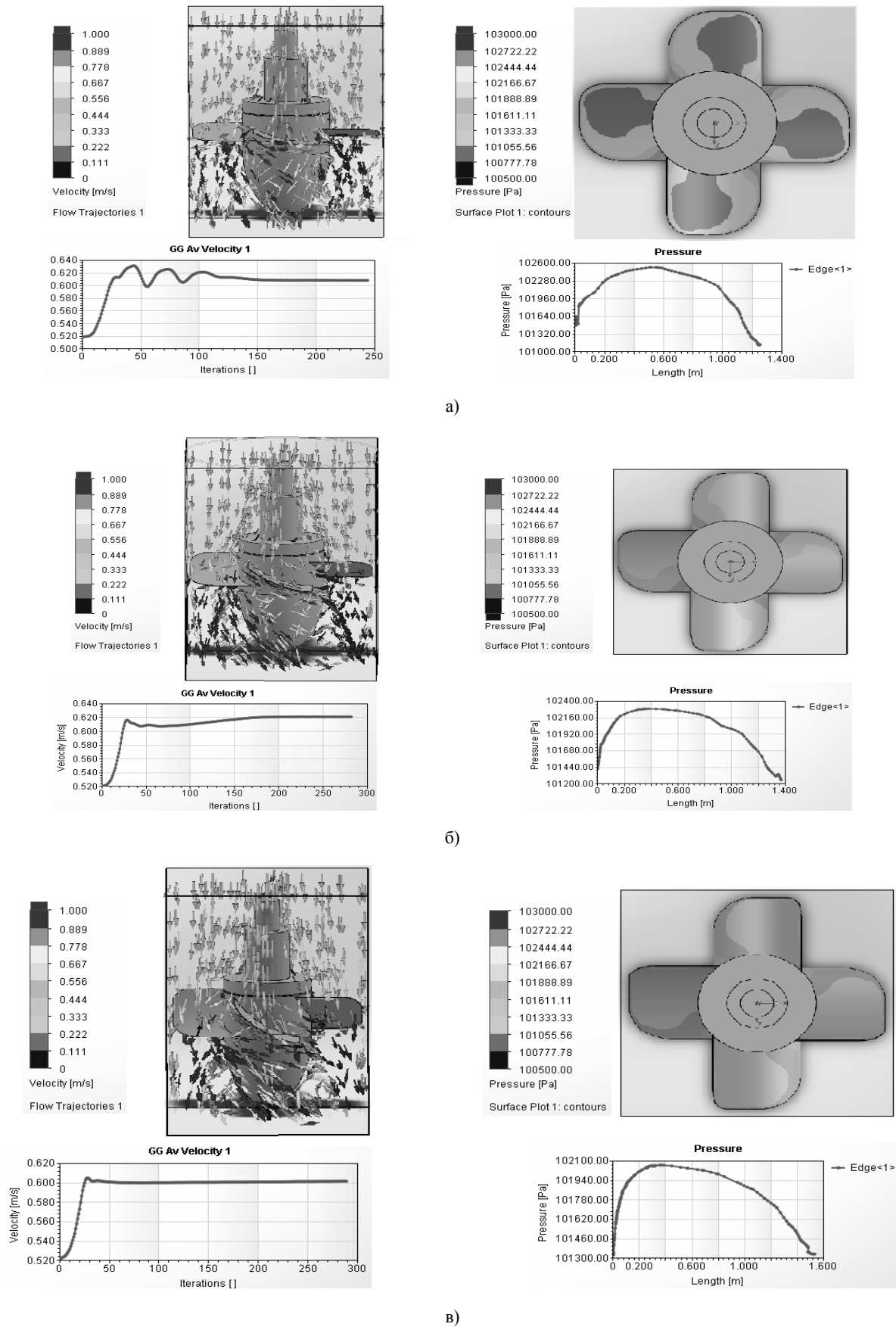
Рис. 4. Розподіл швидкості та тиску на лопаті при різних кутах повороту: а - 15^\circ ; б - 30^\circ ; в - 45^\circ .
