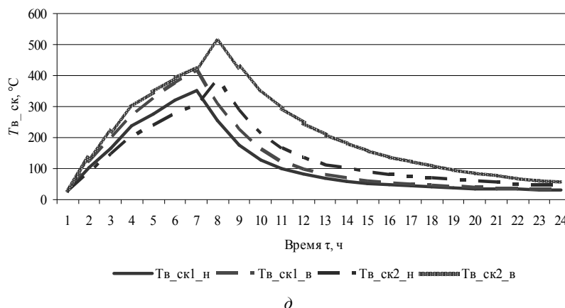
Рис. 2. Результати експериментальних досліджень: а, з – изменение температуры T_{ск} в стенке канала теплоаккумулирующих элементов с каналами прямоугольного сечения и с каналами круглого сечения соответственно в нижней и верхней зоне в течение периода заряда и отдачи теплоты; б, д – изменение температуры нагреваемого воздуха в канале T_{в\_ск} в теплоаккумулирующих элементах с каналами прямоугольного сечения и с каналами круглого сечения соответственно в нижней и верхней зоне в течение периода заряда и отдачи теплоты; в – изменение температуры тепловой изоляции T_{из} в нижней и верхней зоне, на поверхности корпуса T_{с1} и нагретого воздуха на выходе из ЭТА T_{вых} .
