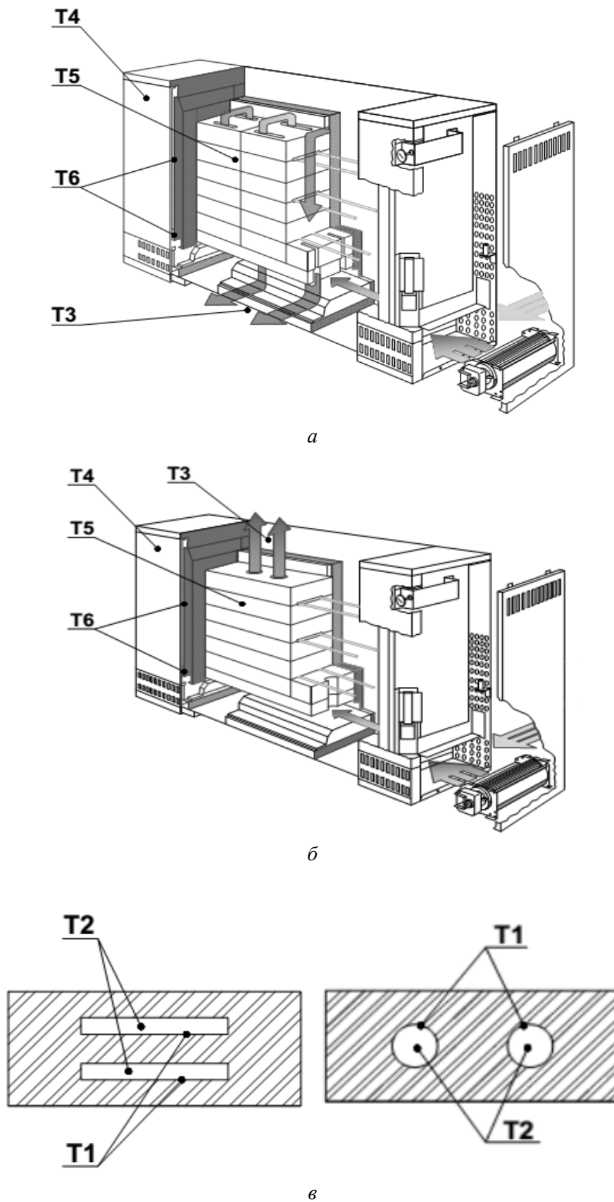
Рис. 1. Схема проведення експерименту по дослідженню динамічних характеристик теплоакumuлюючих елементів ЭТА: а, б – схема ЭТА с теплоакumuлюючими елементами с прямоугольними воздушними каналами (стандартная конструкция) и с каналами круглого сечения с указанием мест установки термопар ТХА; в – места установки термопар ТХА в теплоакumuлюючих элементах в нижней и верхней зоне ЭТА.
