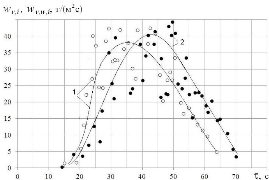
Рис. 3. Поточна швидкість термолізу сухої W_{v,i} та вологої частки W_{v,w,i} деревної гранули діаметром 6 мм при нагріві в окислювальній атмосфері печі при 700 °C: 1 – суха частка; 2 – частка із вмістом води 7,8% мас.
