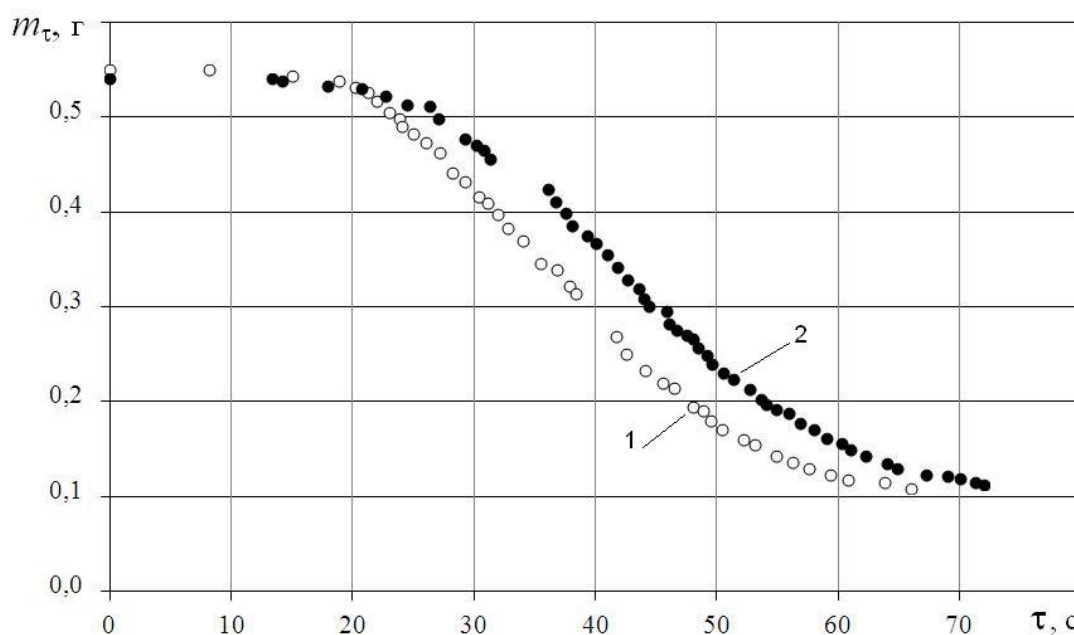
Рис. 1. Зміна маси сухої та вологої часток деревних гранул діаметром 6 мм при термолізі в муфельній печі при 700°C: 1 – суха частка; 2 – частка із вмістом вологи 7,8%.
