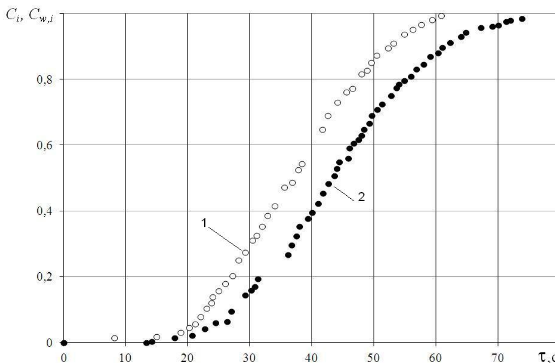
Рис. 2. Динаміка виходу летких із сухої C та водяної пари з леткими C_w з вологої частки деревних гранул в окислювальній атмосфері печі при температурі 700°C: 1 – суха частка; 2 – частка із вмістом води 7,8% мас.
