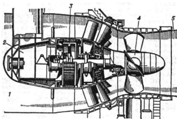
Рис. 3. Горизонтальный капсульный гидроагрегат: 1 – подводящая камера; 2 – капсула; 3 – гидрогенератор; 4 – рабочее колесо гидротурбины; 5 – отсасывающая труба.
