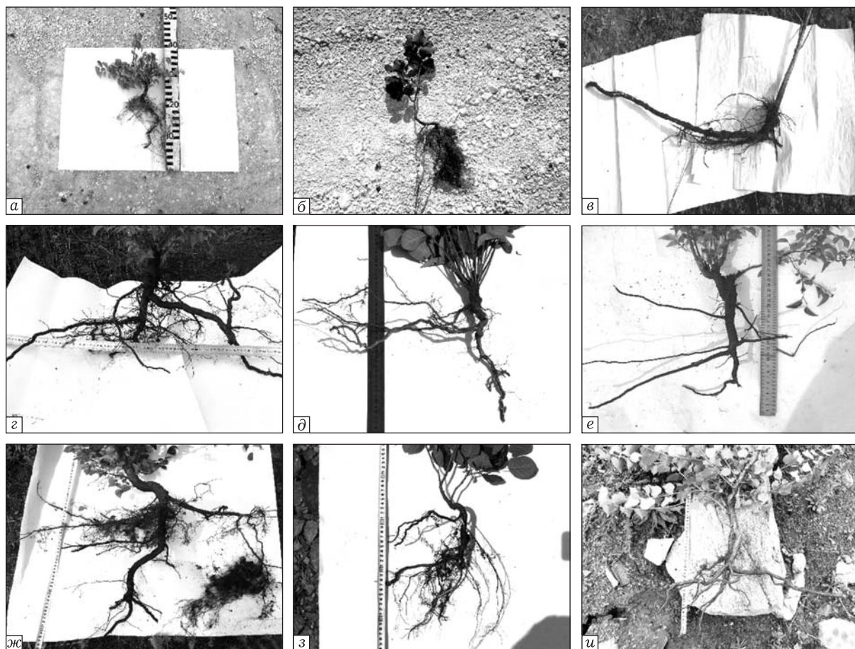
Морфоструктура корневой системы древесных растений на меловых отвалах содового производства, терриконах угольных шахт Донбасса и железорудных отвалах Криворожья: а — Padellus mahaleb на меловых отвалах; б — Cotinus coggigia на меловых отвалах; в — Armeniaca vulgaris на меловых отвалах; г — Padellus mahaleb на железорудных отвалах; д — Cotinus coggigia на железорудных отвалах; е — Armeniaca vulgaris на железорудных отвалах; ж — Padellus mahaleb на угольных терриконах; з — Cotinus coggigia на угольных терриконах; и — Armeniaca vulgaris на угольных терриконах
